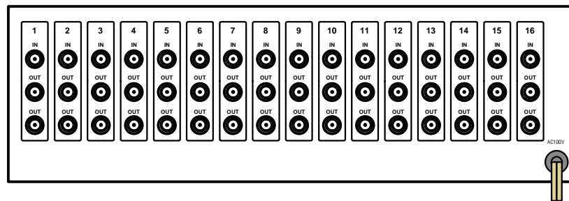
映像分配器（2分配16系統）
