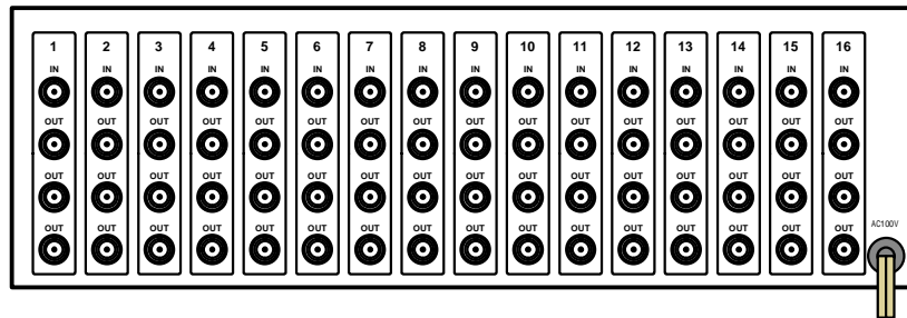
映像分配器（3分配16系統）
